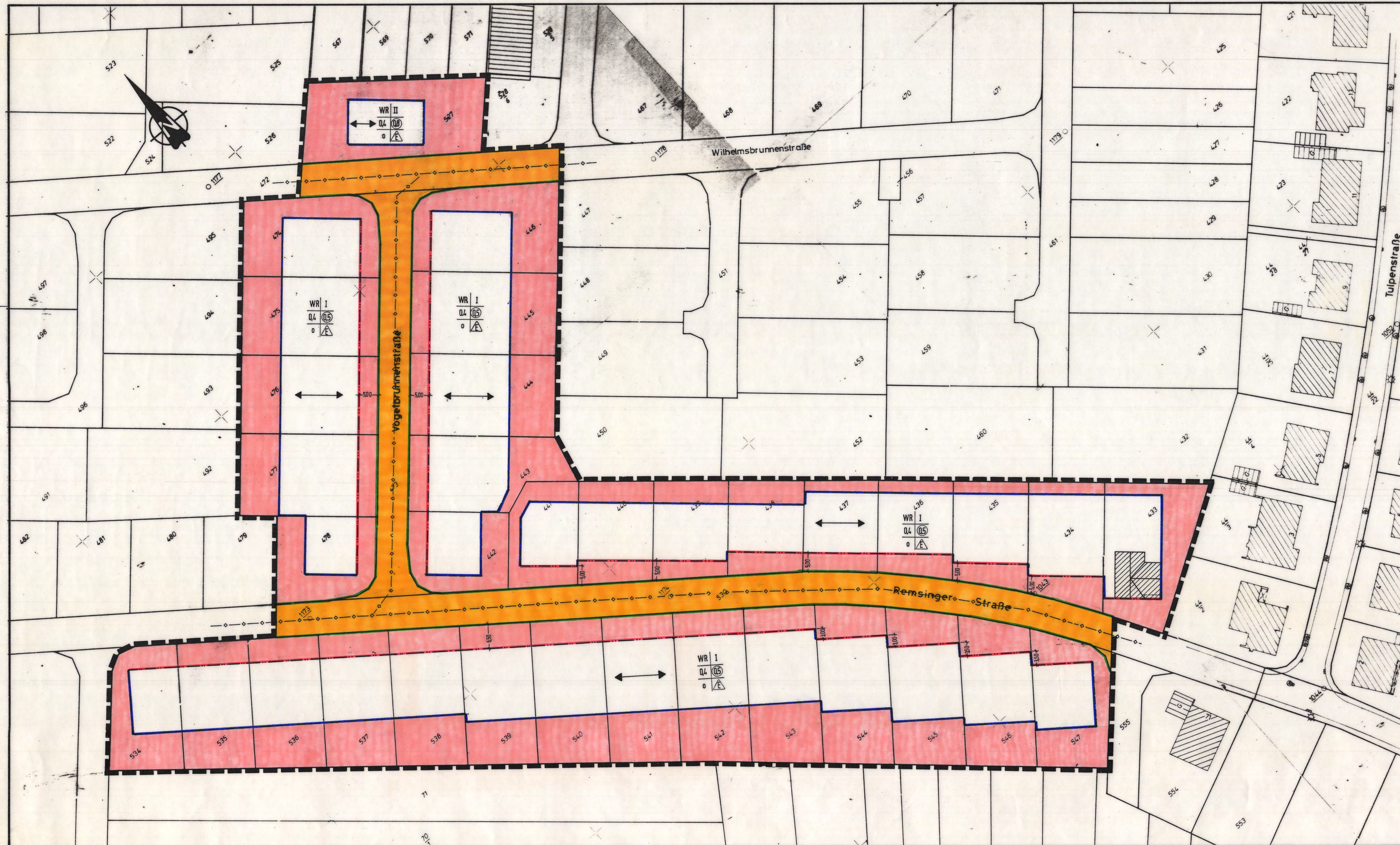
1:500 Genehmigung des Landesvermessungsamtes des Saarlandes vom 01.08.1986, Kontrollnr. B / 004 / 86
